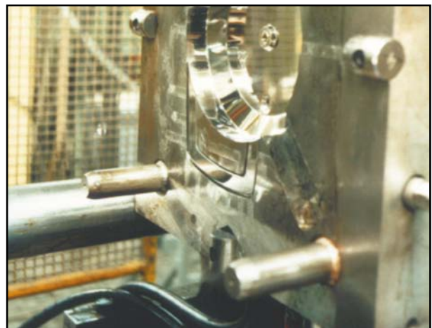
移动旋转线盘的模具, 选择618HH材料
